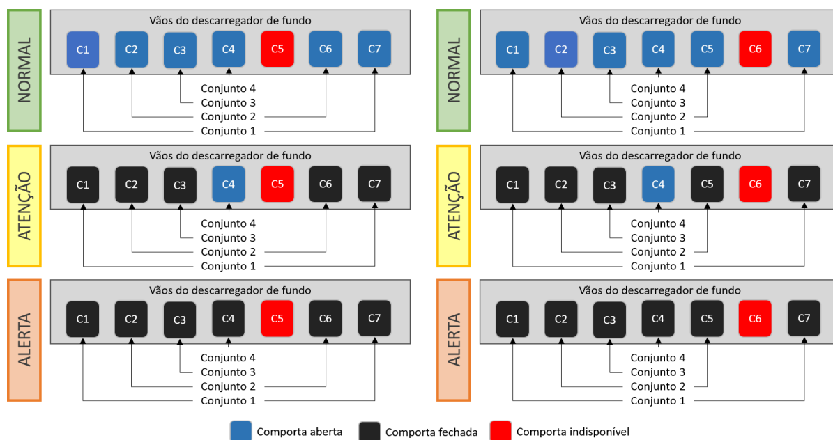
Figura 55. Dinâmica de fechamento das comportas da barragem Oeste em caso de indisponibilidade das comportas C5 ou C6.
