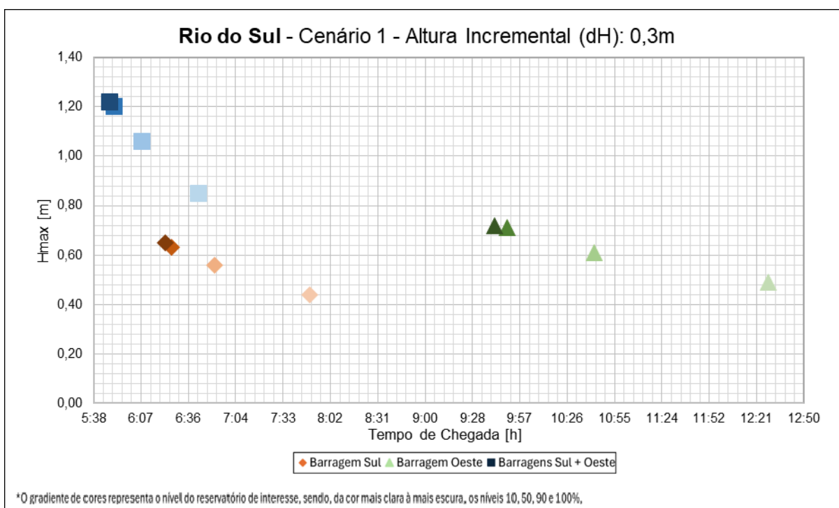
Figura 43. Análise do tempo de chegada e altura incremental para o cenário hidrológico 1 – Rio do Sul –comportas de fundo e canal lateral.
