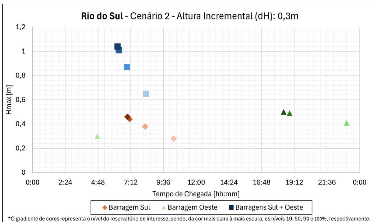
Figura 44. Análise do tempo de chegada e altura incremental para o cenário hidrológico 2 – Rio do Sul – apenas comportas de fundo.
