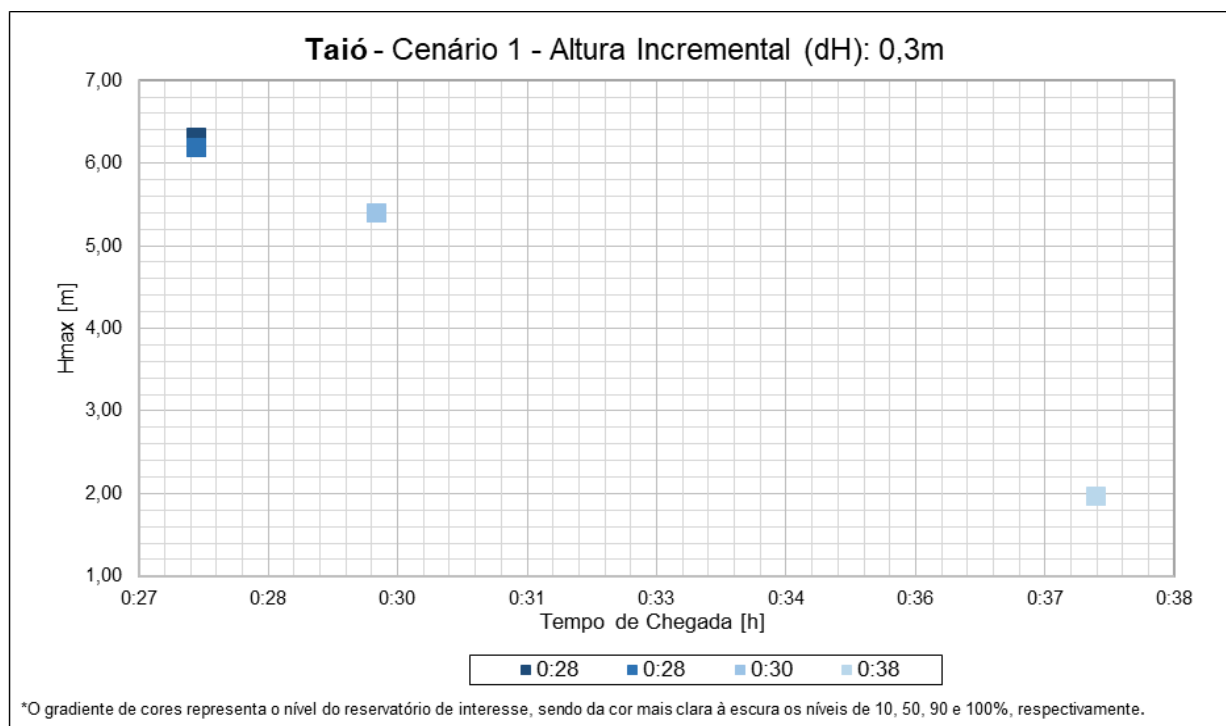
Figura 31. Análise do tempo de chegada e altura incremental para o cenário hidrológico 1 – Taió –comportas de fundo e canal lateral.
