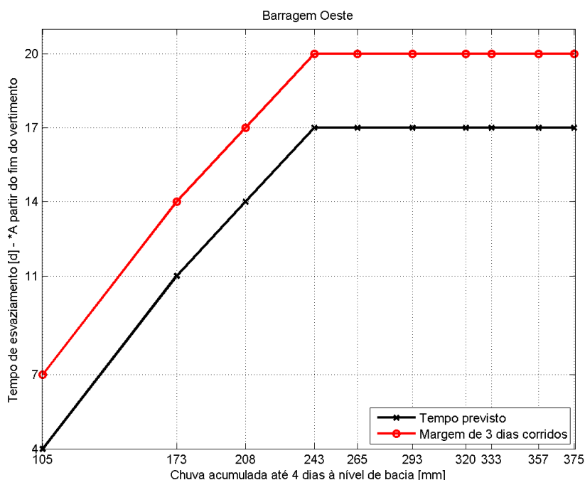
Figura 16. Tempos de esvaziamento da Barragem Oeste.
