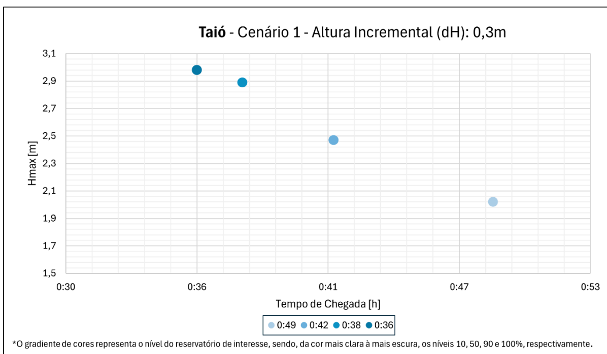
Figura 30. Análise do tempo de chegada e altura incremental para o cenário hidrológico 1 – Taió – apenas comportas de fundo.
