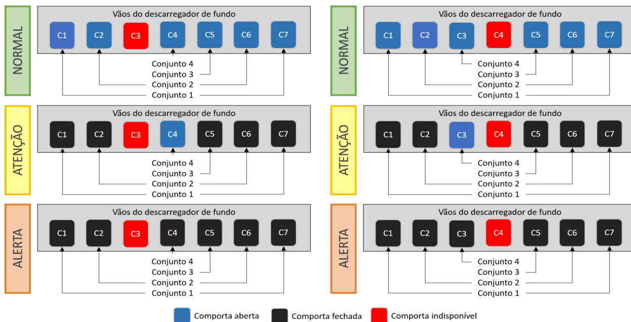
Figura 54. Dinâmica de fechamento das comportas da barragem Oeste em caso de indisponibilidade das comportas C3 ou C4.
