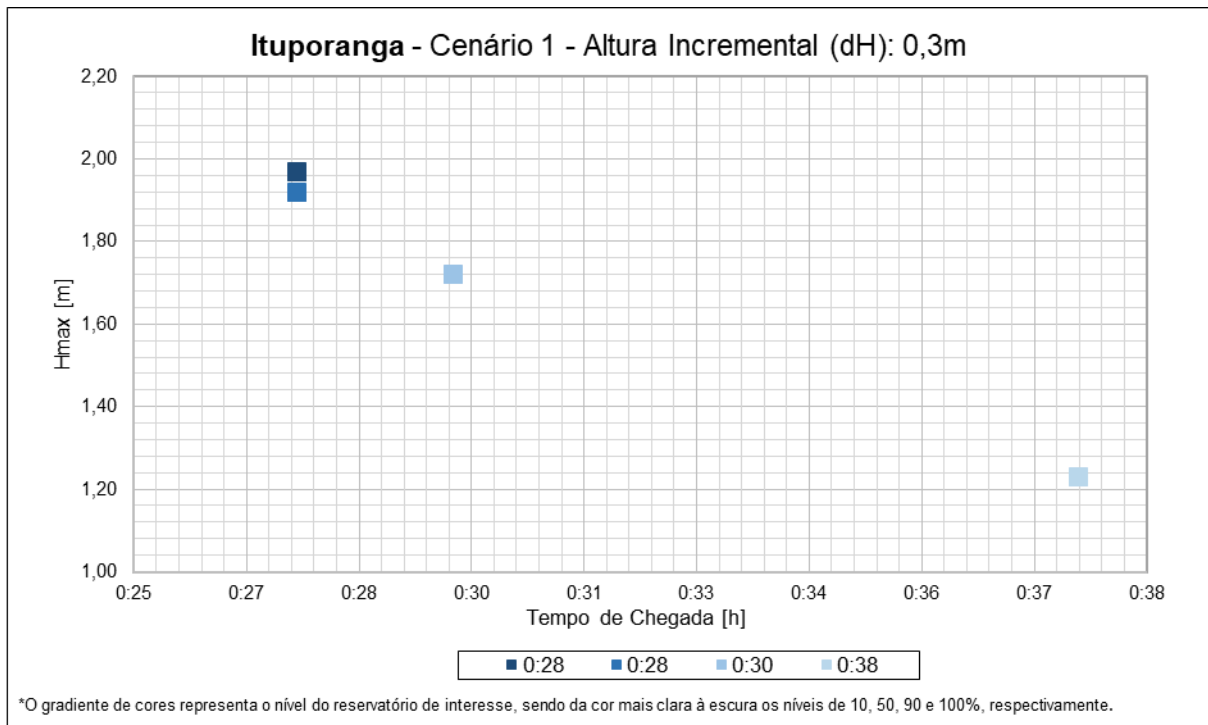
Figura 25. Análise do tempo de chegada e altura incremental para o cenário hidrológico 1 – Ituporanga –comportas de fundo e canal lateral.
