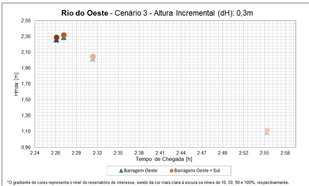
Figura 41. Análise do tempo de chegada e altura incremental para o cenário hidrológico 3 – Rio do Oeste –comportas de fundo e canal lateral.
