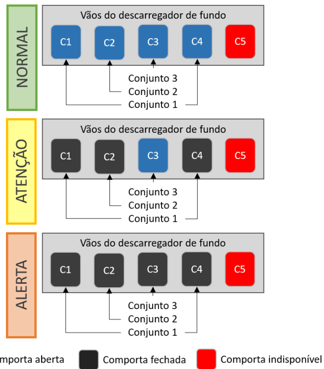
Figura 52. Dinâmica de fechamento das comportas da barragem Sul em caso de indisponibilidade da comporta C5.
