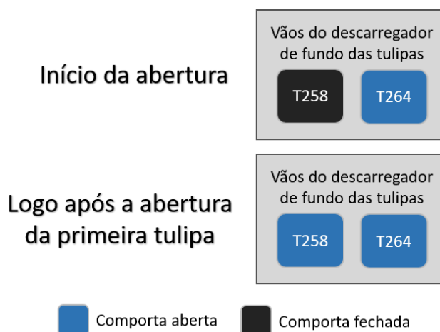
Figura 20. Dinâmica de abertura das comportas das tulipas para o processo de esvaziamento do reservatório da Barragem Norte.
