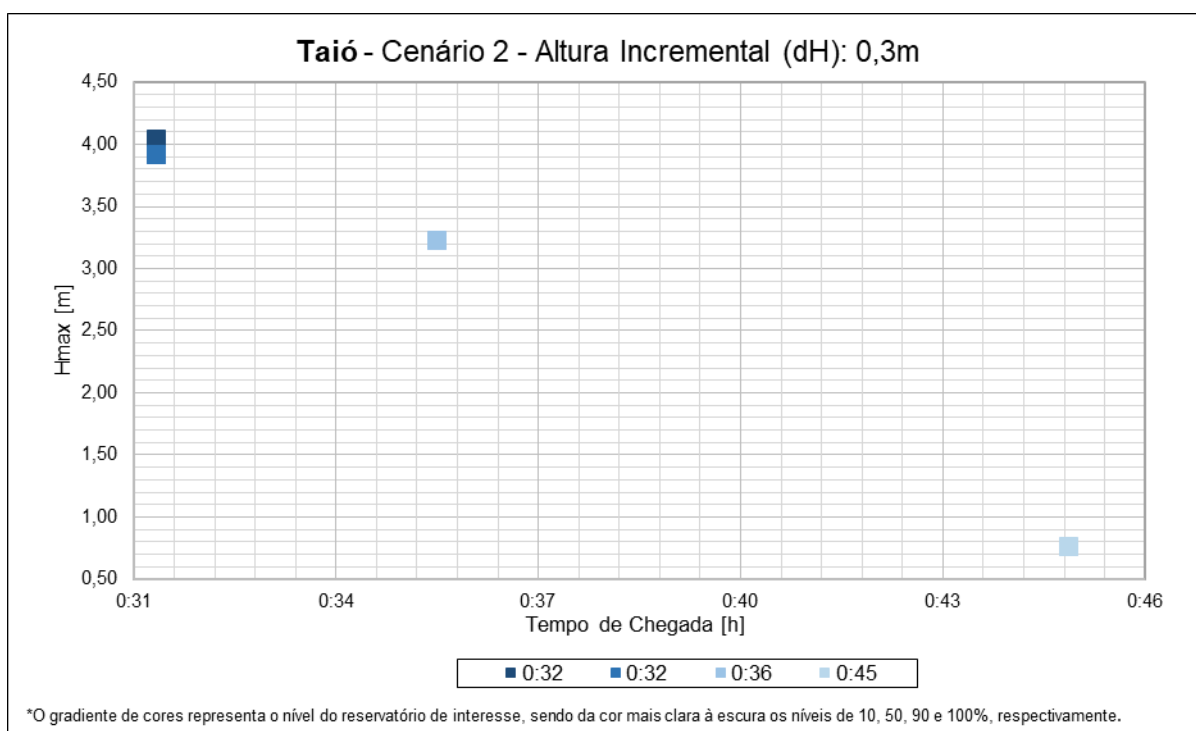
Figura 33. Análise do tempo de chegada e altura incremental para o cenário hidrológico 2 – Taió –comportas de fundo e canal lateral.
