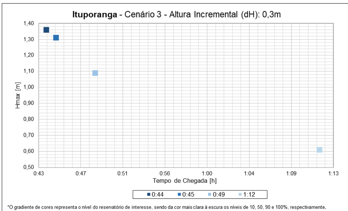
Figura 29. Análise do tempo de chegada e altura incremental para o cenário hidrológico 3 – Ituporanga –comportas de fundo e canal lateral.
