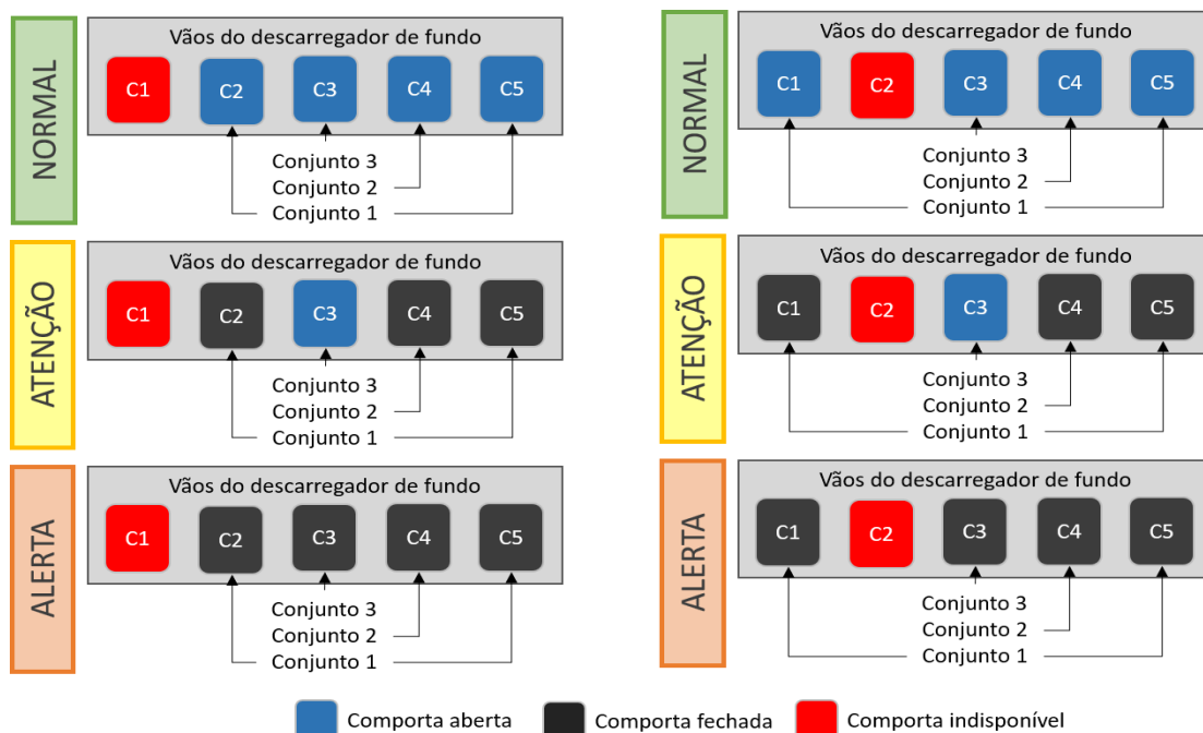
Figura 50. Dinâmica de fechamento das comportas da barragem Sul em caso de indisponibilidade das comportas C1 ou C2.
