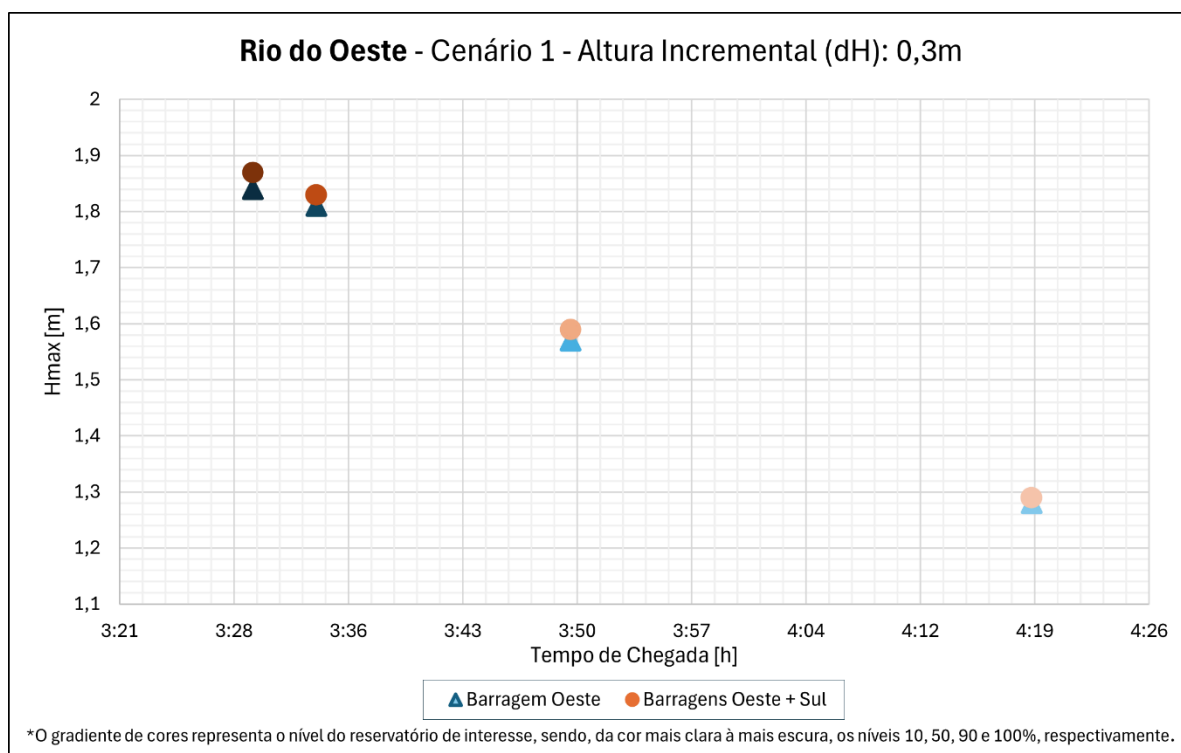
Figura 36. Análise do tempo de chegada e altura incremental para o cenário hidrológico 1 – Rio do Oeste – apenas comportas de fundo.
