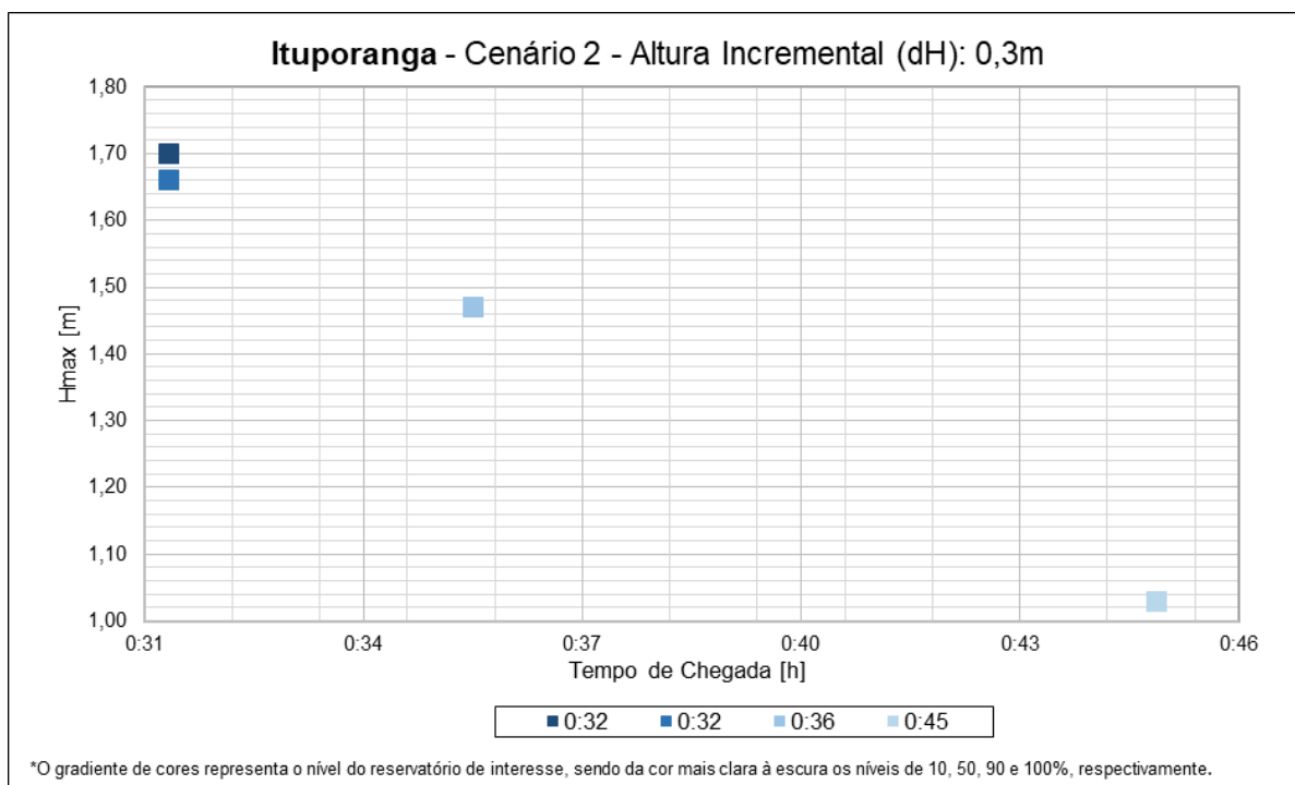
Figura 27. Análise do tempo de chegada e altura incremental para o cenário hidrológico 2 – Ituporanga –comportas de fundo e canal lateral.
