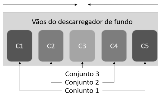
Figura 4. Dinâmica das comportas do descarregador de fundo – Barragem Sul.
