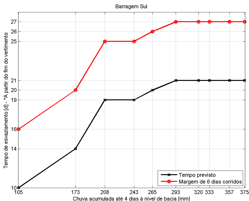
Figura 13. Tempo de esvaziamento da Barragem Sul.
