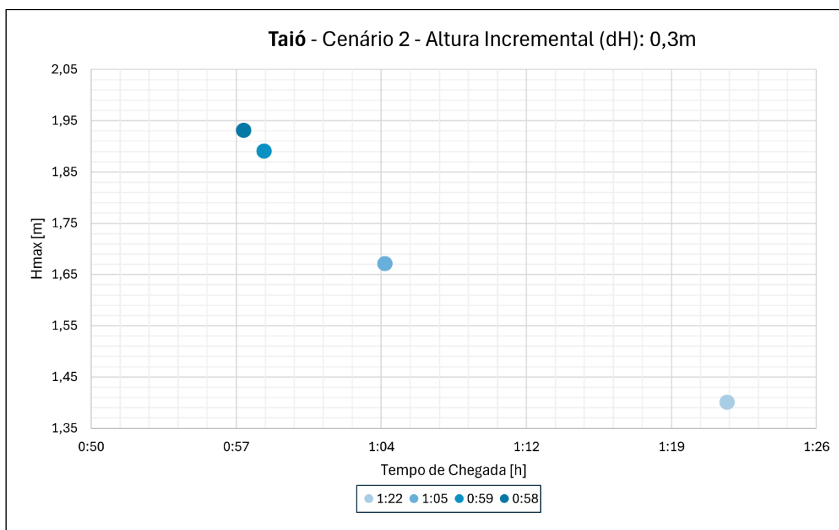
Figura 32. Análise do tempo de chegada e altura incremental para o cenário hidrológico 2 – Taió – apenas comportas de fundo.
