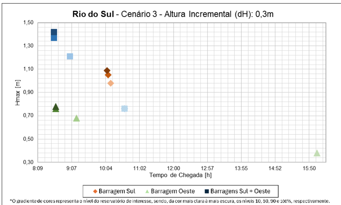
Figura 47. Análise do tempo de chegada e altura incremental para o cenário hidrológico 3 – Rio do Sul –comportas de fundo e canal lateral.
