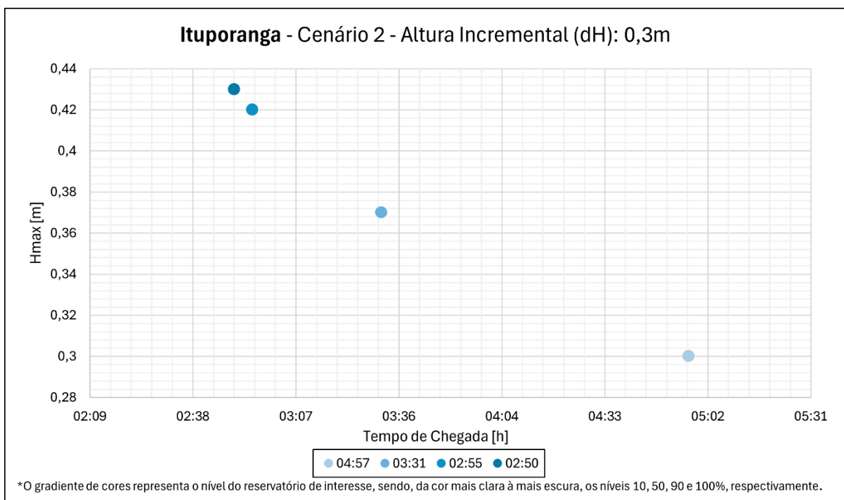
Figura 26. Análise do tempo de chegada e altura incremental para o cenário hidrológico 2 – Ituporanga– apenas comportas de fundo.
