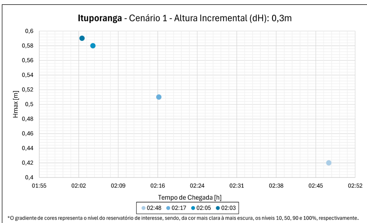
Figura 24. Análise do tempo de chegada e altura incremental para o cenário hidrológico 1 – Ituporanga – apenas comportas de fundo.
