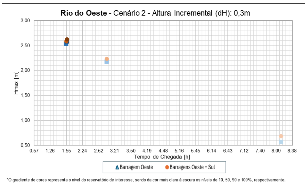
Figura 39. Análise do tempo de chegada e altura incremental para o cenário hidrológico 2 – Rio do Oeste –comportas de fundo e canal lateral.
