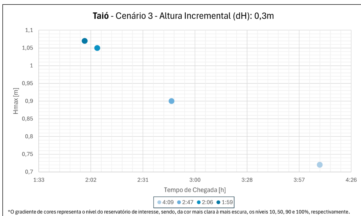
Figura 34. Análise do tempo de chegada e altura incremental para o cenário hidrológico 3 – Taió – apenas comportas de fundo.
