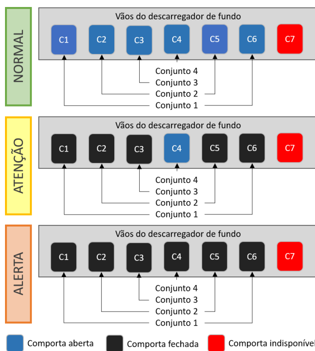
Figura 56. Dinâmica de fechamento das comportas da barragem Oeste em caso de indisponibilidade da comporta C7.
