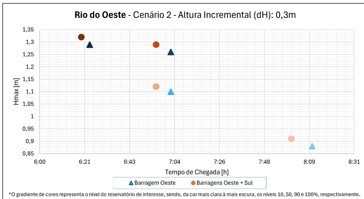
Figura 38. Análise do tempo de chegada e altura incremental para o cenário hidrológico 2 – Rio do Oeste – apenas comportas de fundo.
