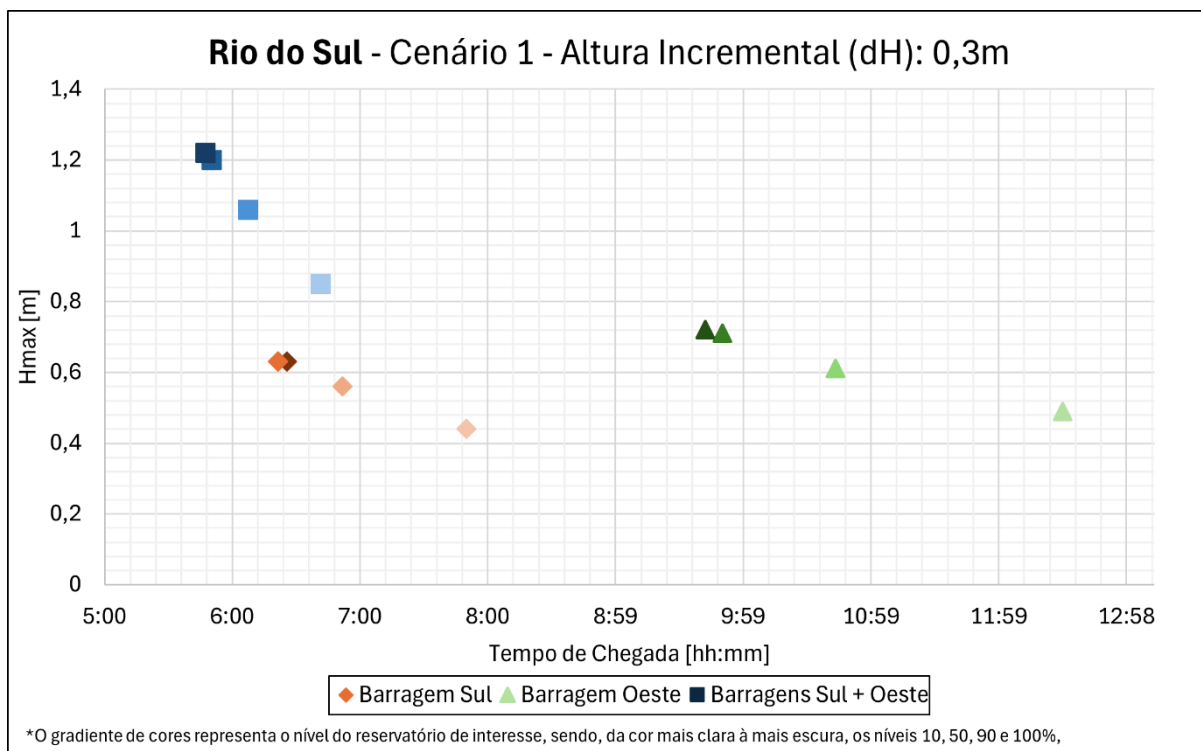
Figura 42. Análise do tempo de chegada e altura incremental para o cenário hidrológico 1 – Rio do Sul – apenas comportas de fundo.
