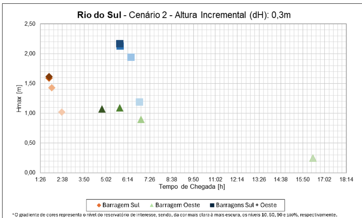
Figura 45. Análise do tempo de chegada e altura incremental para o cenário hidrológico 2 – Rio do Sul –comportas de fundo e canal lateral.
