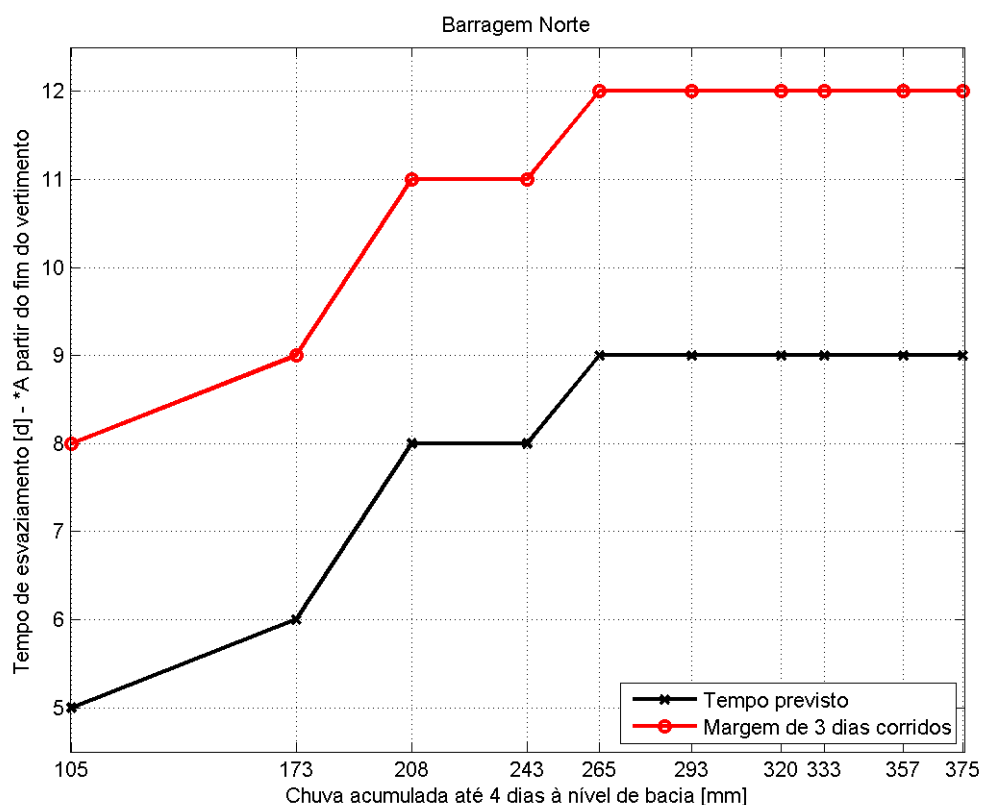
Figura 19. Tempo de esvaziamento da Barragem Norte.
