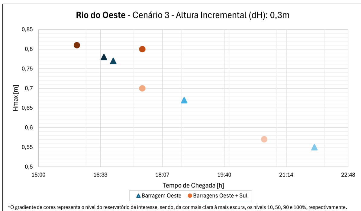
Figura 40. Análise do tempo de chegada e altura incremental para o cenário hidrológico 3 – Rio do Oeste – apenas comportas de fundo.
