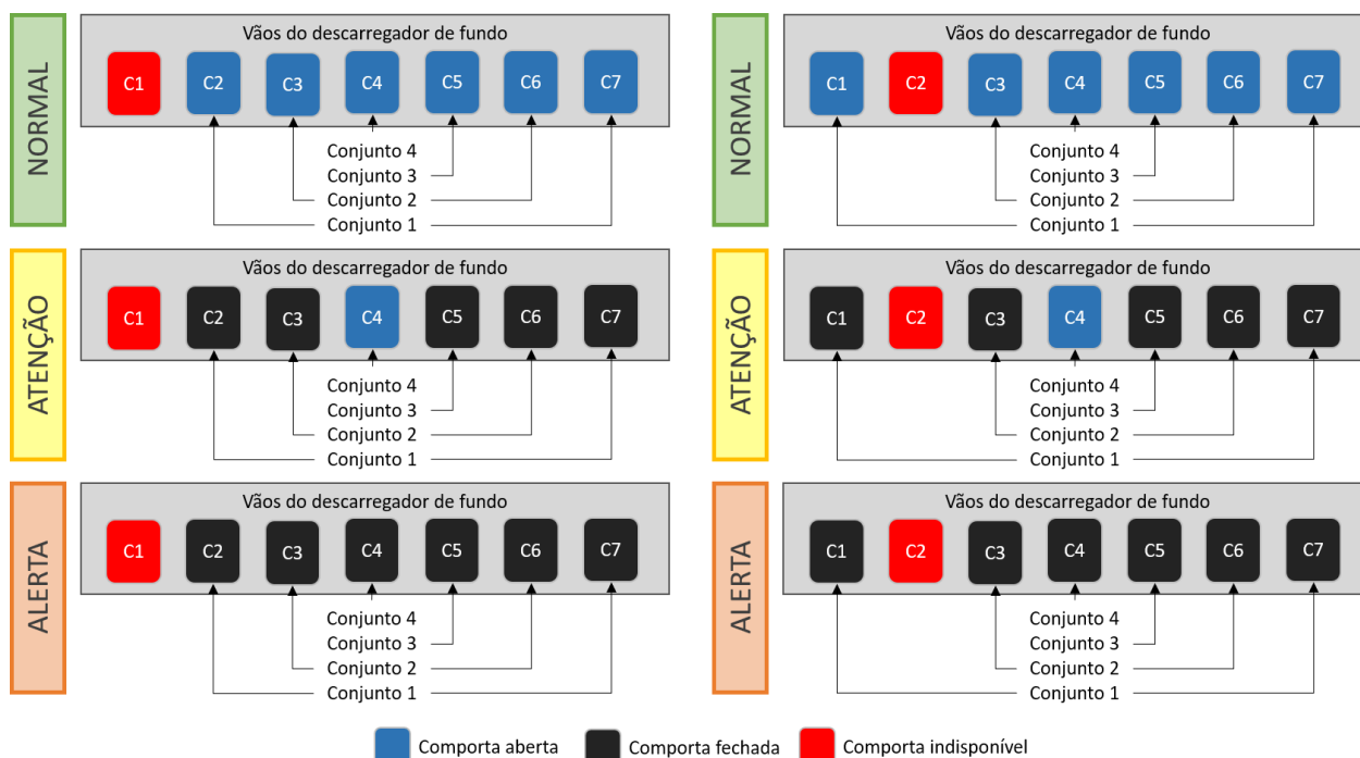
Figura 53. Dinâmica de fechamento das comportas da barragem Oeste em caso de indisponibilidade das comportas C1 ou C2.
