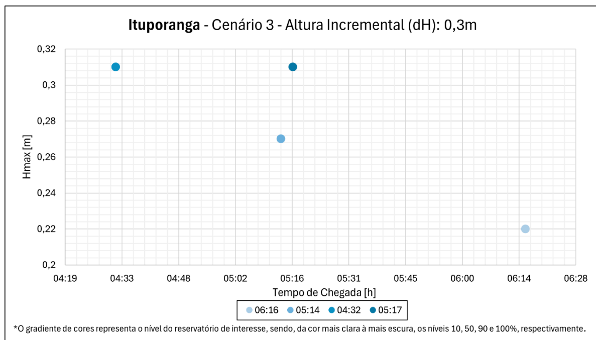
Figura 28. Análise do tempo de chegada e altura incremental para o cenário hidrológico 3 – Ituporanga – apenas comportas de fundo.
