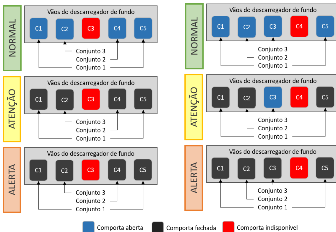
Figura 51. Dinâmica de fechamento das comportas da barragem Sul em caso de indisponibilidade das comportas C3 ou C4.
