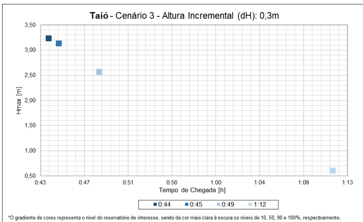
Figura 35. Análise do tempo de chegada e altura incremental para o cenário hidrológico 3 – Taió –comportas de fundo e canal lateral.
