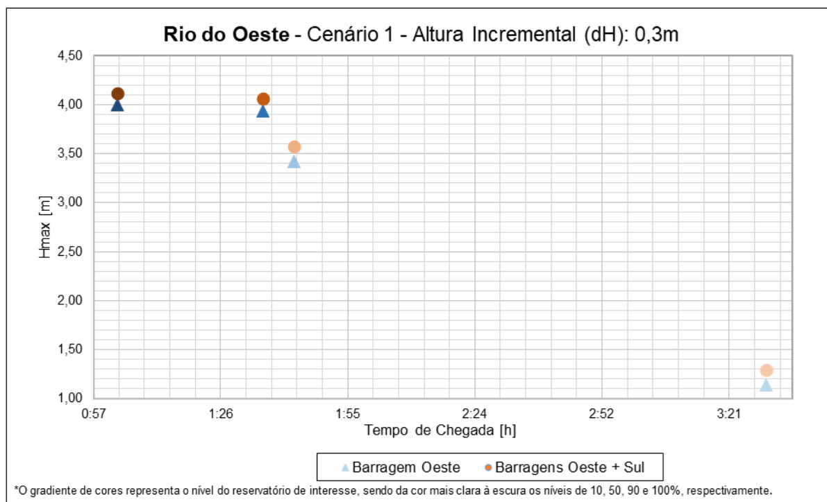
Figura 37. Análise do tempo de chegada e altura incremental para o cenário hidrológico 1 – Rio do Oeste –comportas de fundo e canal lateral.
