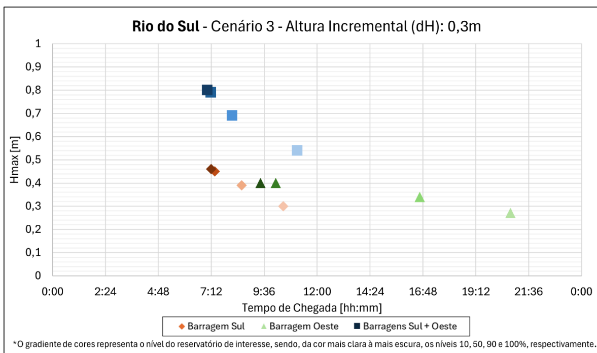
Figura 46. Análise do tempo de chegada e altura incremental para o cenário hidrológico 3 – Rio do Sul – apenas comportas de fundo.
